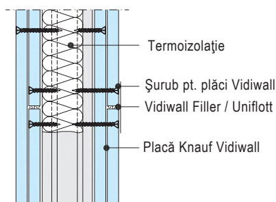
W362-VM1-A Îmbinarea orizontală
