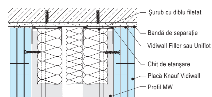
W345-V01-A Racord la tavan
