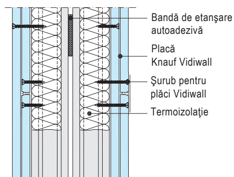
W365-VM1-A Îmbinarea orizontală
