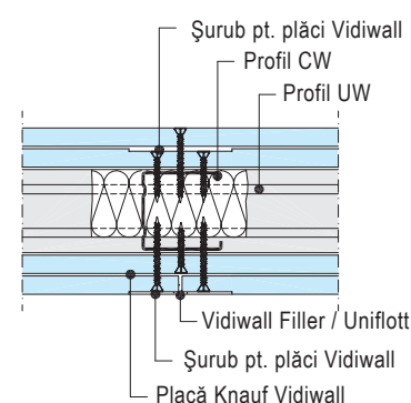
W362-B1 Îmbinarea plăcilor
