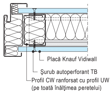
W361-E2-A Realizarea golului de ușă cu profile CW/UW
