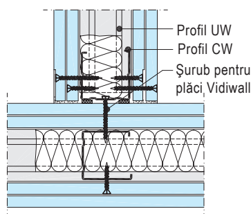
W362-C1 Îmbinare în T
