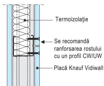
W361-VM1-A Îmbinarea orizontală
