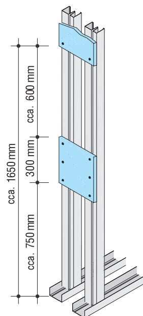
Ranforsarea scheletului metalic cu ștraifuri Vidiwall ≥ 12.5 mm grosime și 300 mm lățime
