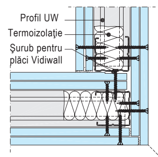
W362-D1 Realizarea colțurilor
