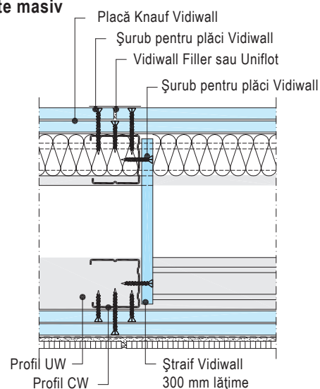
W366-D1 Joncțiune cu W112
