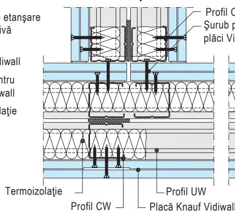
W365-C1 Îmbinare în T
