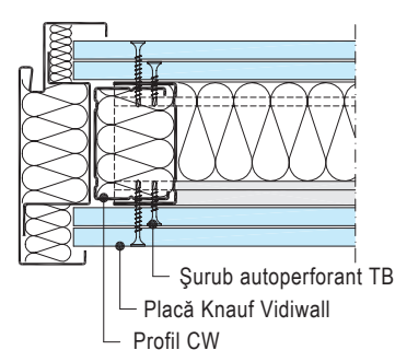
W362-E2-A Realizarea golului de ușă cu profile CW/UW
