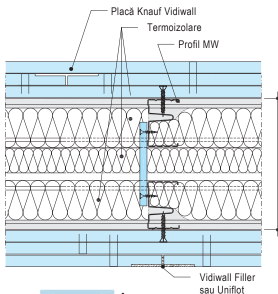
W361-B1 Îmbinarea plăcilor
