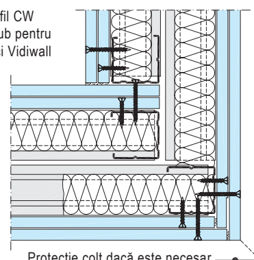
W365-B1 Îmbinarea plăcilor
