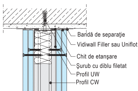
W362-V01-A Racord la tavan
